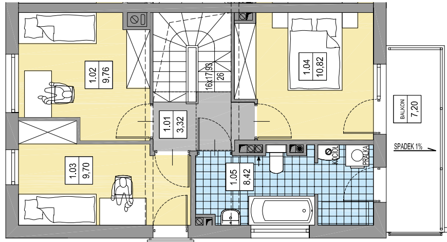
RZUT PIĘTRA
