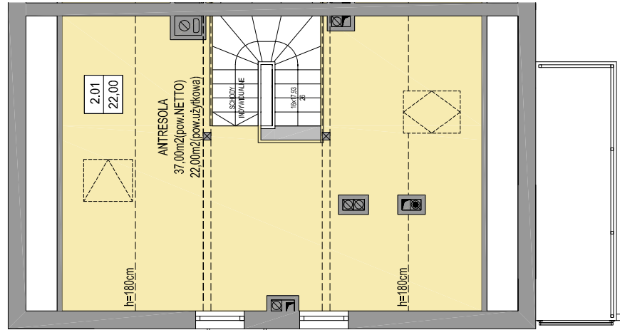
RZUT ANTRESOLI
