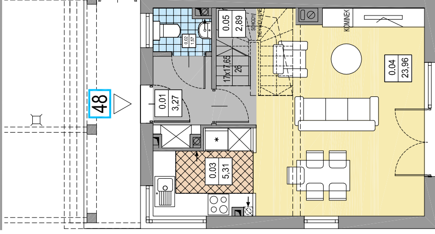
RZUT PARTERU
