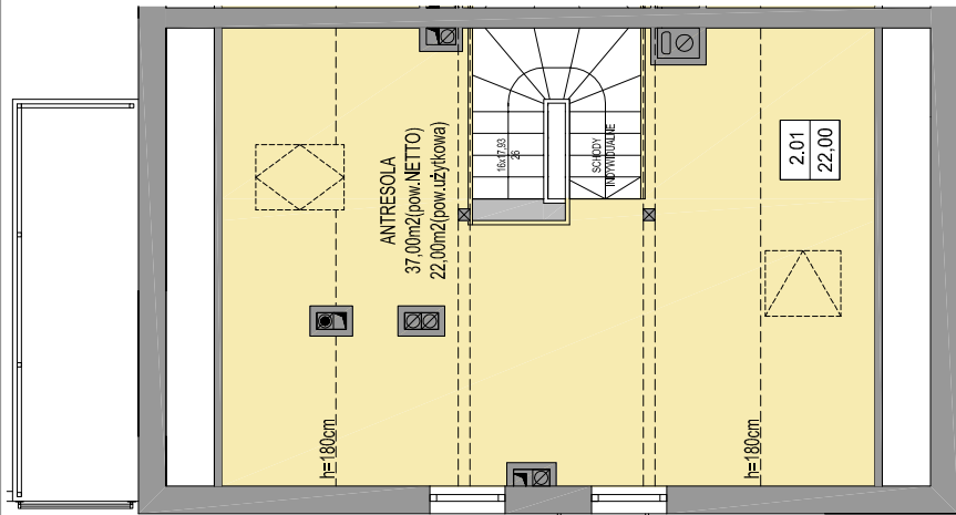
RZUT ANTRESOLI
