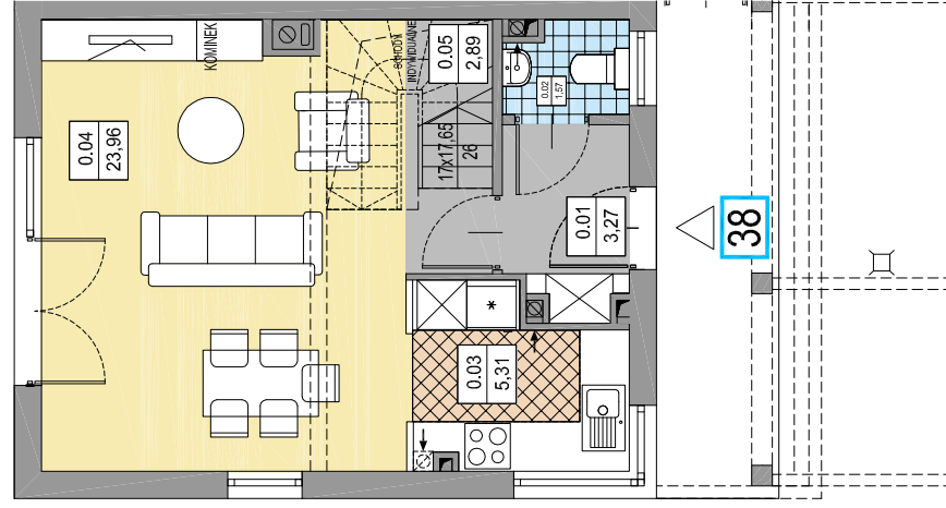
RZUT PARTERU
