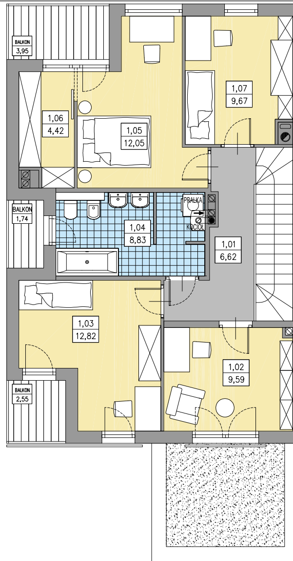
RZUT PIĘTRA
