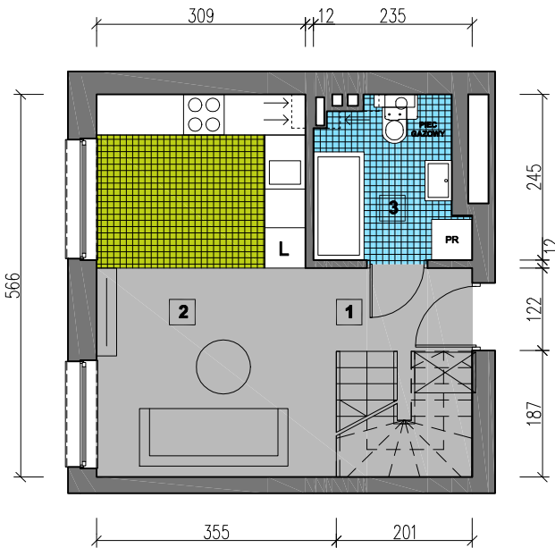
POZIOM 1
